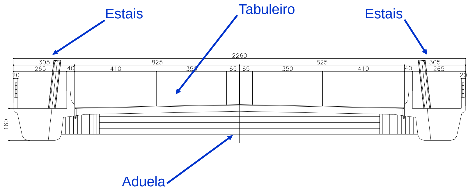
Seção Transversal do Tabuleiro no Trecho Estaiado
