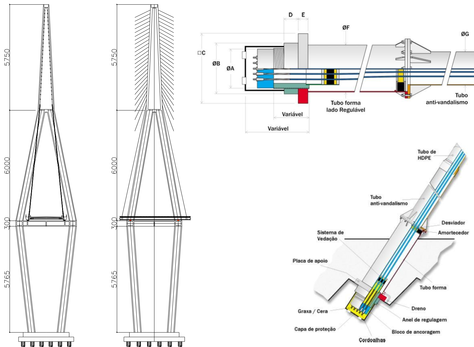
Detalhes do Mastro Central em forma de diamante e da fixação dos Estais
