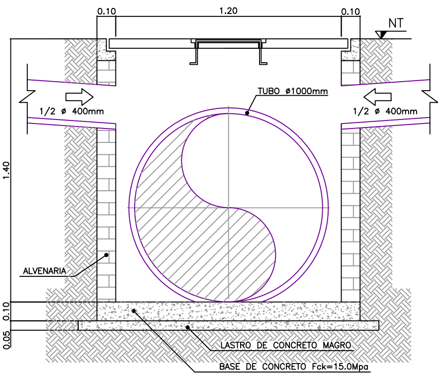
CORTE EE
