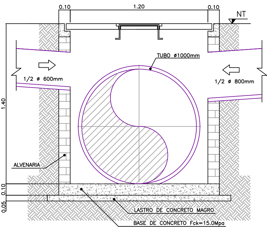
CORTE DD
