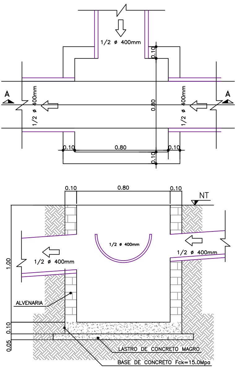
CAIXA DE PASSAGEM PARA CANALETA Ø 400 mm
