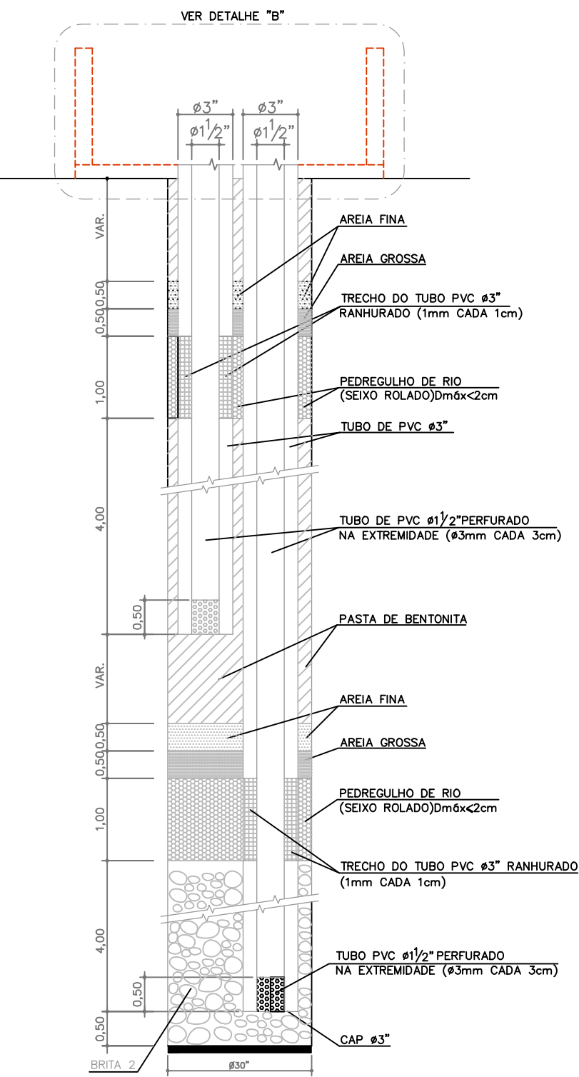
DETALHE DO PIEZÔMETRO DE 2 CÂMARAS
