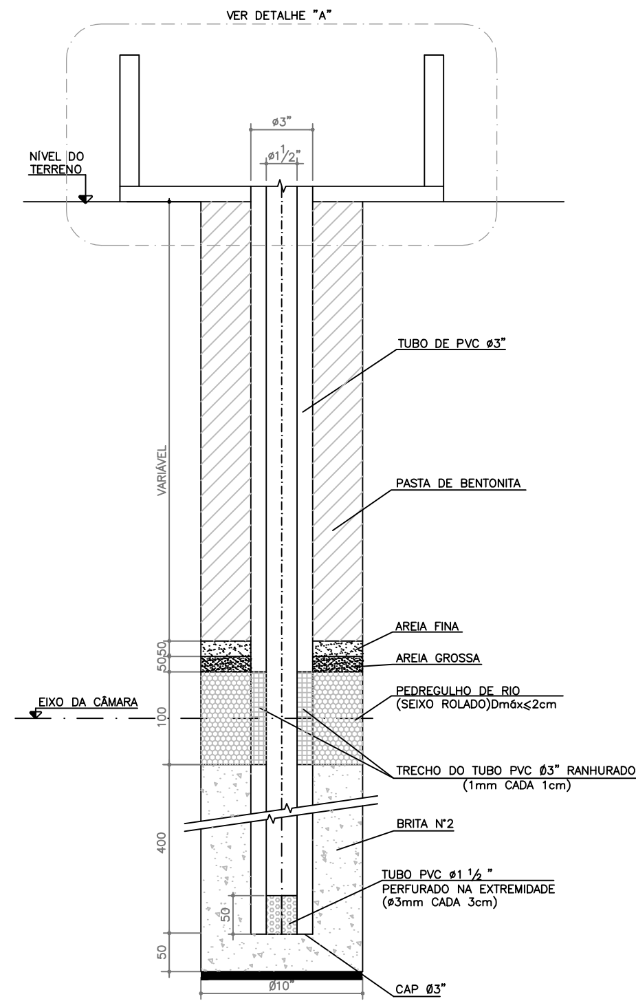
DETALHE DO PIEZÔMETRO DE 1 CÂMARA
